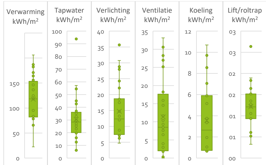
Figuur 3. Spreiding (boxplot) van het energieverbruik per m 2 BVO van de zes belangrijkste energiegebruikende processen in een zorglocatie.
