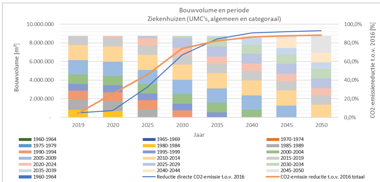
Figuur 13. Resultaten doelscenario 4, maatregelenpakket B: bouwvolume, periode (kwaliteit gebouwschil) en CO 2 -emissiereductie t.o.v. 2016
