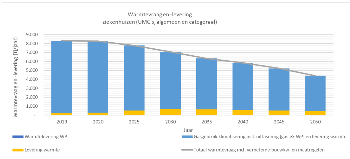
Figuur 12. Resultaten doelscenario 2, maatregelenpakket A: Ontwikkeling warmtevraag en -levering (warmtepompen en aansluiting op warmtenet)
