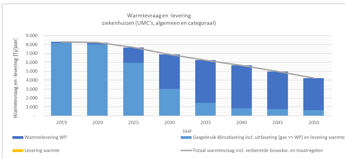
Figuur 17. Resultaten doelscenario 4, maatregelenpakket B: Ontwikkeling warmtevraag en -levering (warmtepompen en aansluiting op warmtenet)
