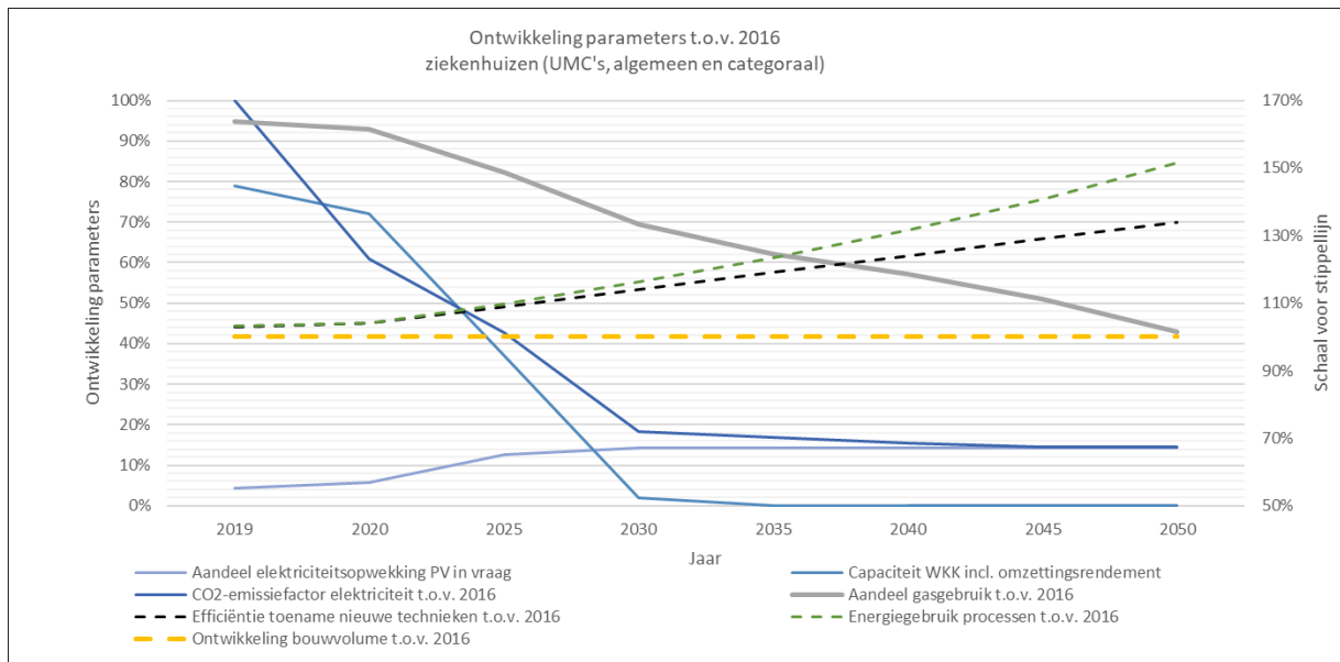
Figuur 11. Resultaten doelscenario 2, maatregelenpakket A: Ontwikkeling parameters t.o.v. 2016 (op basis van gelijkblijvend bouwvolume (m 2 ) volgens gele stippellijn)
