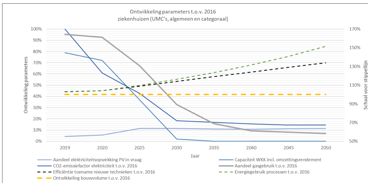
Figuur 16. Resultaten doelscenario 4, maatregelenpakket B: Ontwikkeling parameters t.o.v. 2016 (op basis van gelijkblijvend bouwvolume (m 2 ) volgens gele stippelijijn)
