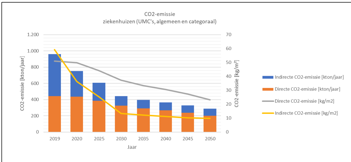
Figuur 10. Resultaten doelscenario 2, maatregelenpakket A: jaarlijkse CO 2 -emissie (absoluut en per m 2 )
