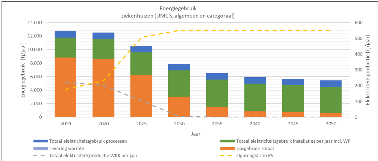
Figuur 14. Resultaten doelscenario 4, maatregelenpakket B: energiegebruik en elektriciteitsproductie (opbrengst PV-zonnepanelen) per jaar
