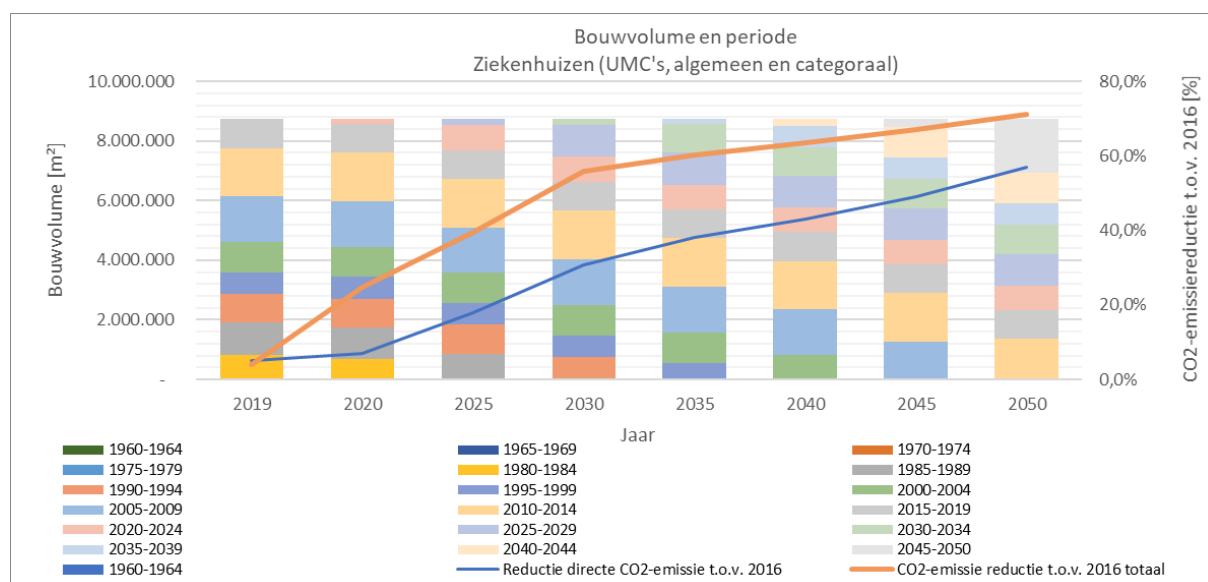
Figuur 8. Resultaten doelscenario 2, maatregelenpakket A: bouwvolume, periode (kwaliteit gebouwschil) en CO 2 -emissiereductie t.o.v. 2016
