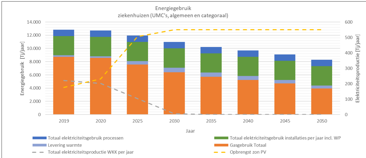
Figuur 9. Resultaten doelscenario 2, maatregelenpakket A: energiegebruik en elektriciteitsproductie (opbrengst PV-zonnepanelen) per jaar
